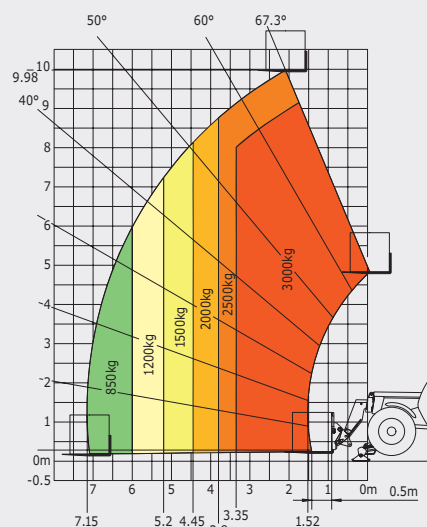
ДИАГРАММА НАГРУЗКИ для внедорожных условий согласно норме EN 1459 B
